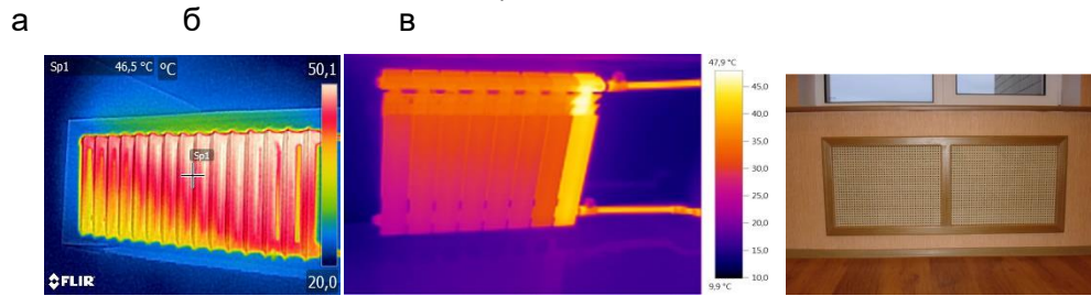
Рис. 3. Термограми роботи опалювальних приладів: а – рівномірна тепловіддача в ідеальному опалювальному приладі; б – більша частина опалювального приладу не віддає тепло (дефект монтажу секцій); в – опалювальний прилад закритий декоративними решітками і має недостатню тепловіддачу
